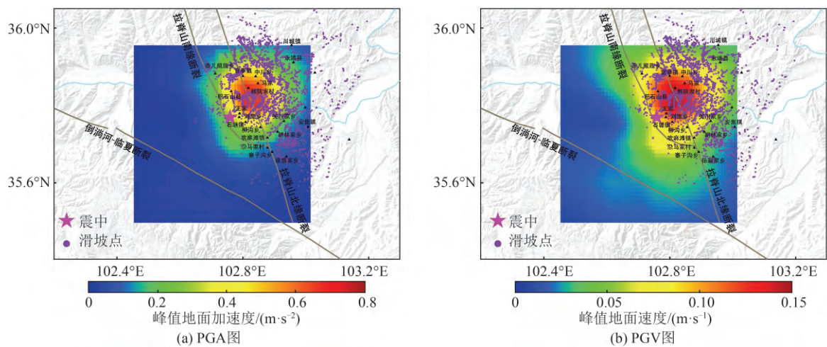
图 6 PGA 图和 PGV 图 Fig. 6 PGA Map and PGV Map
