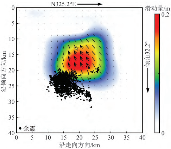
图3 同震滑动分布模型
