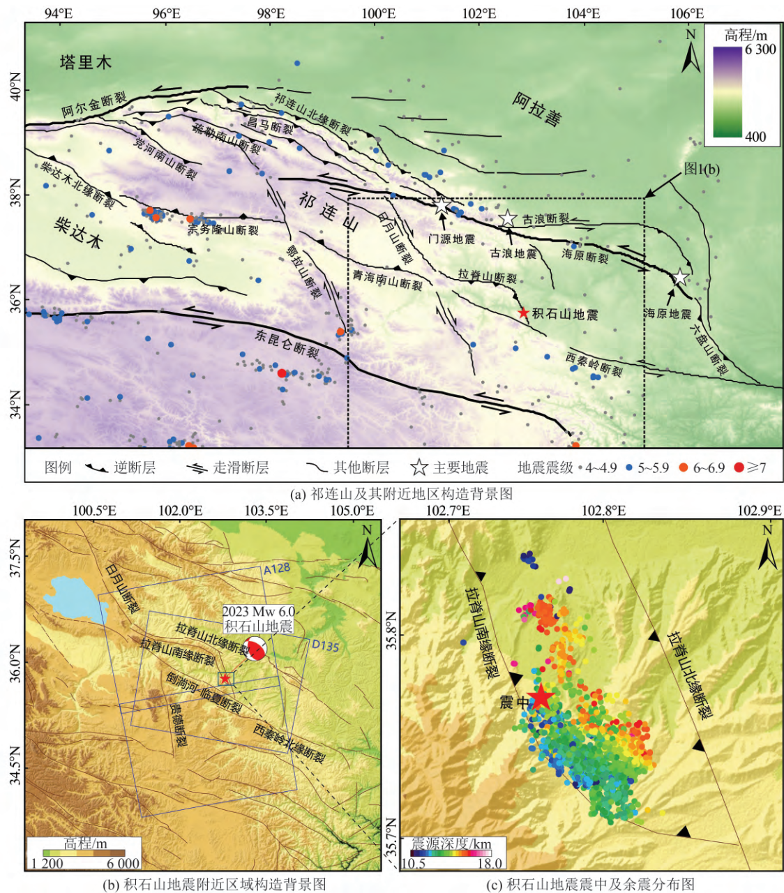
图 1 青藏高原东北缘构造背景及积石山地震附近区域构造图
