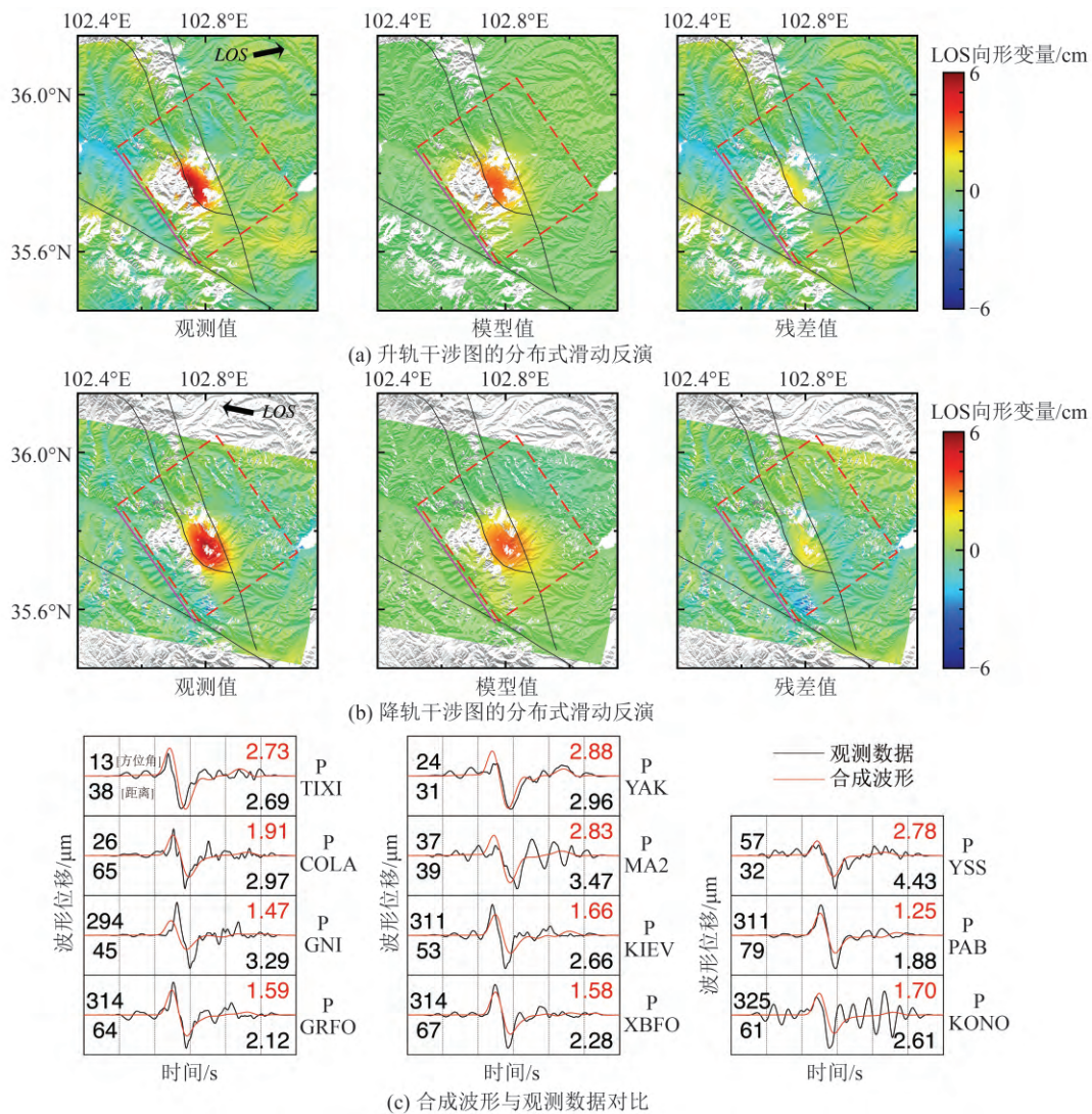
图4 滑动分布反演观测值、模型值及残差值
