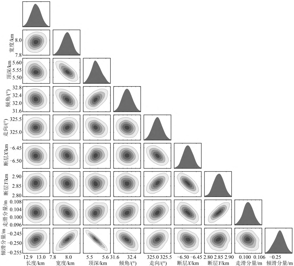
图2 断层几何参数联合概率密度分布图
